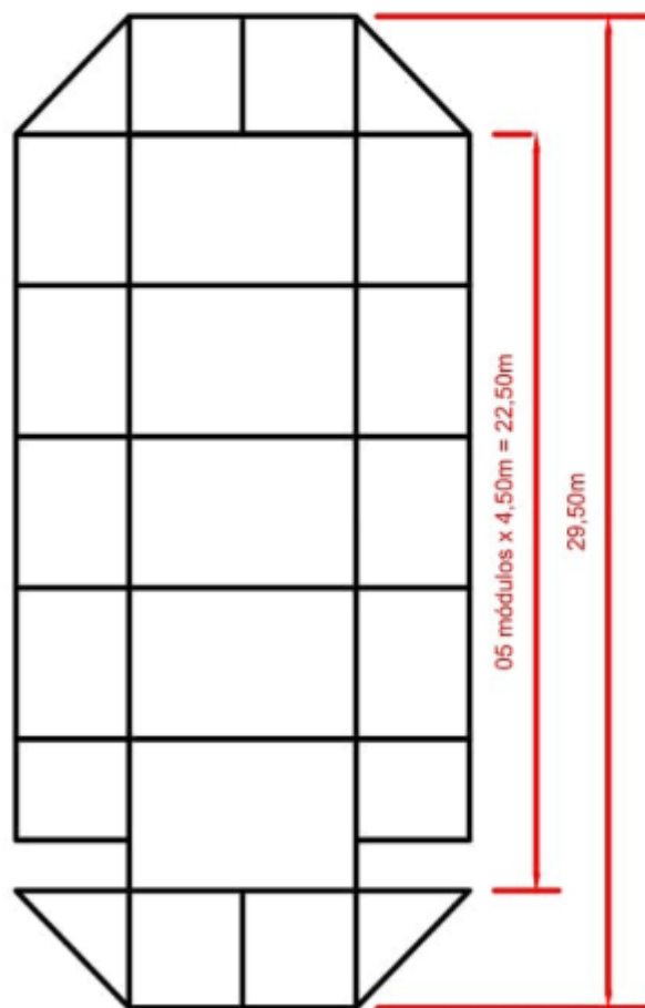
Planta baixa
